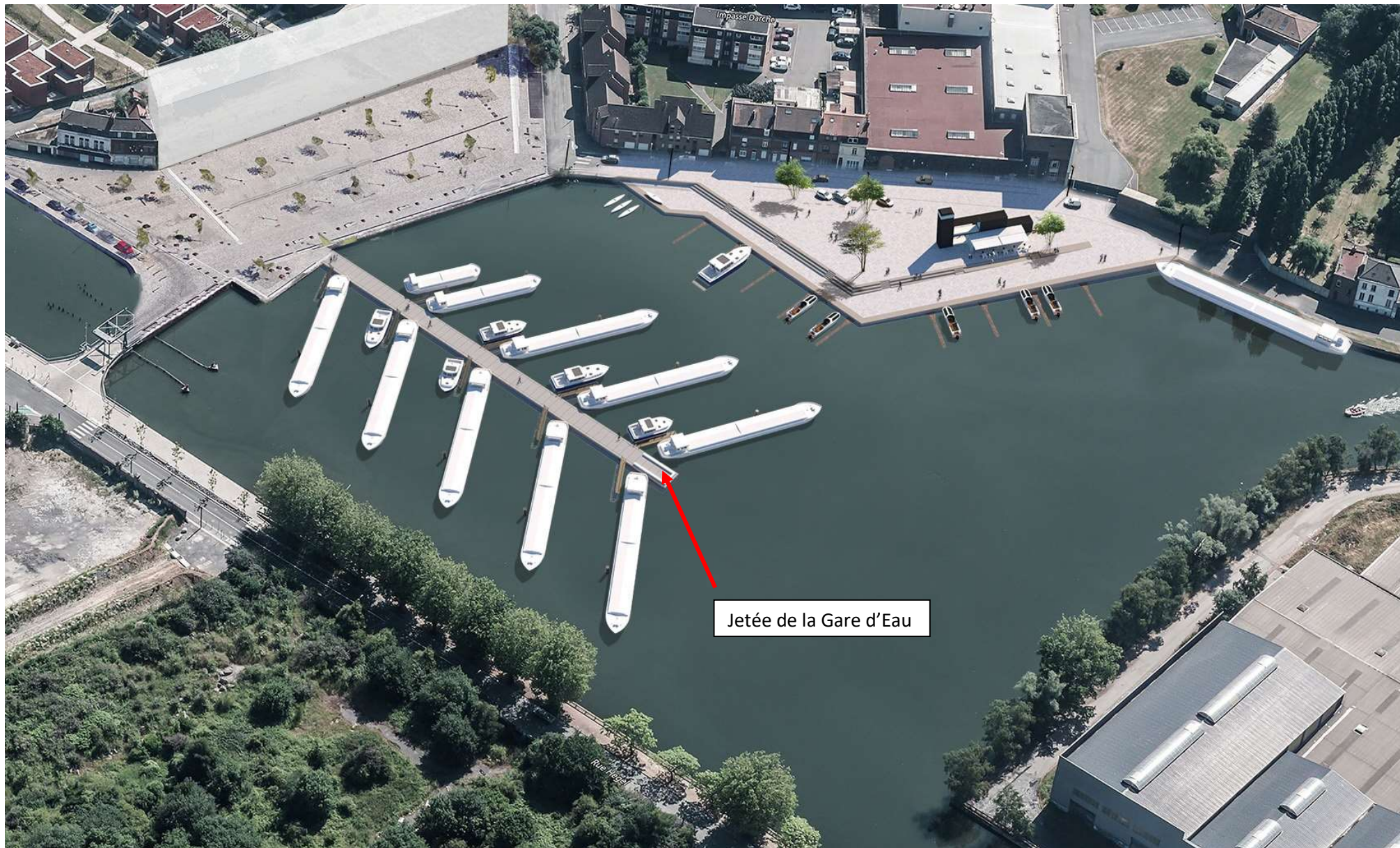
Requalification de la Gare d'Eau : insertion en état futur.
